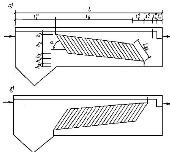
Рисунок -3. Схема отстойника, оборудованного тонкослойными блоками, работающего па противоточной схеме удаления примесей:
