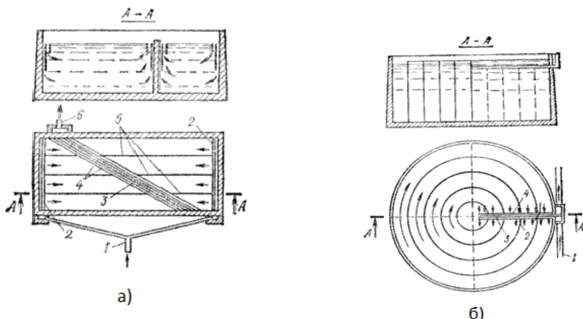
Рисунок - 1 Прямоугольный усреднитель (а) и круглый (б) концентрации сточных вод:
