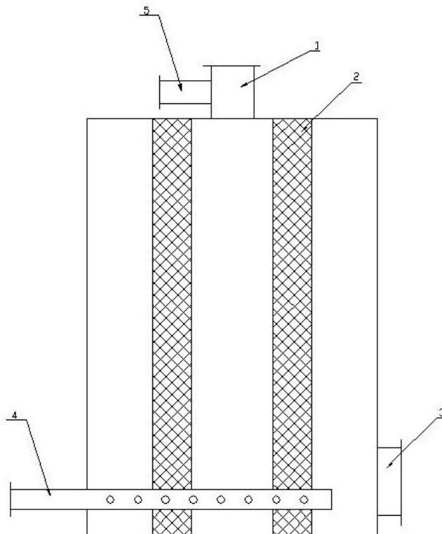
Рис. 4. Адсорбер вертикальный:
