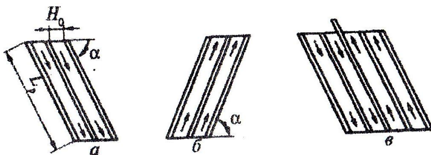
Рис. 2. Расположение полочных и трубчатых элементов в тонкослойных отстойниках:
