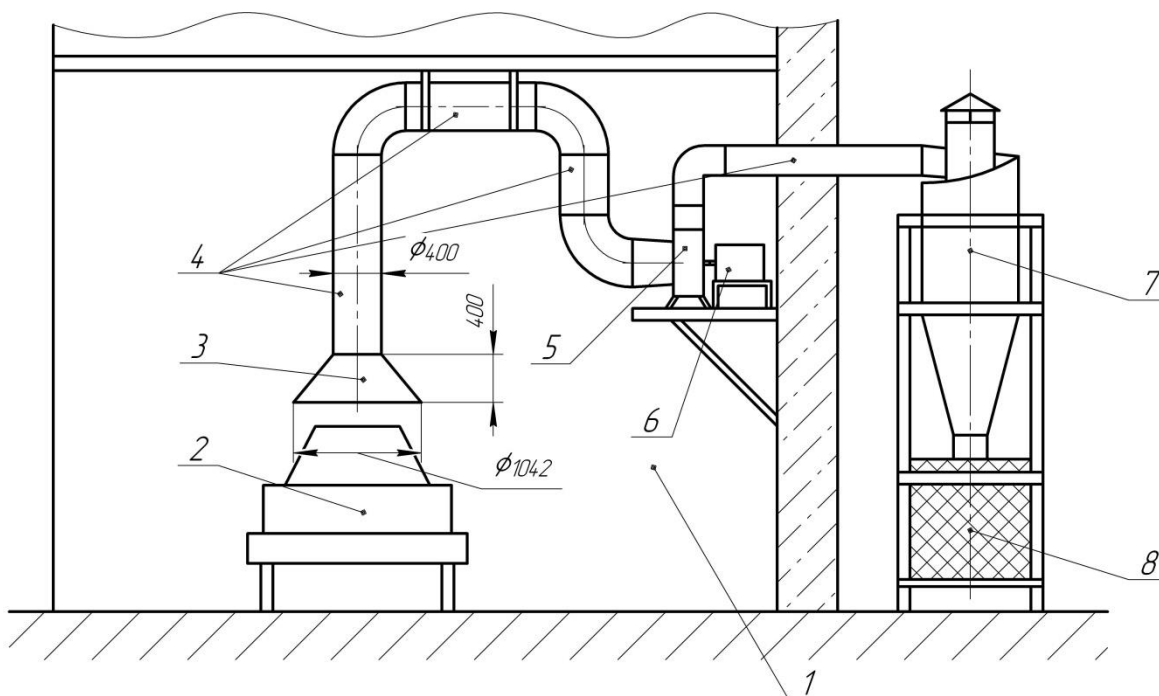
Рисунок 1 – Расчетная схема вентиляции
