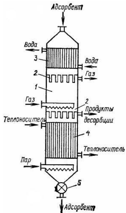
Рис. 2. Адсорбер с движущимся слоем адсорбента:
