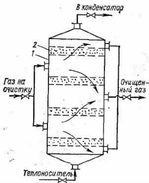
Рис. 1. Адсорбер полочного типа с неподвижными слоями адсорбента:
